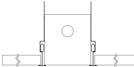
LT9 - 9/16 LAY-IN
